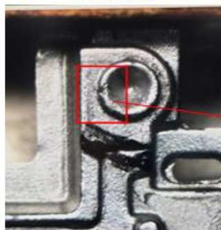
비산으로 인한 보스 형상부 미성형 발생
