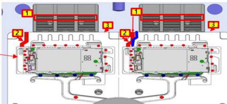
비산방지과 미성형 개선위한 금형디자인 개선
